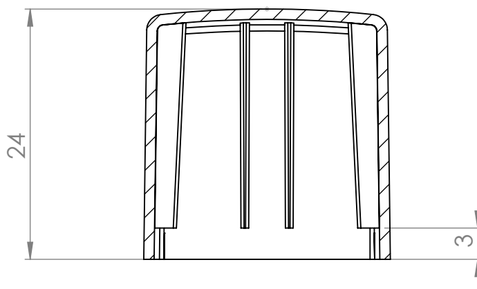
PRZEKRÓJ A-A
