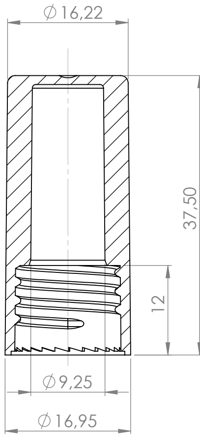
PRZEKRÓJ A-A SKALA 2 : 1
